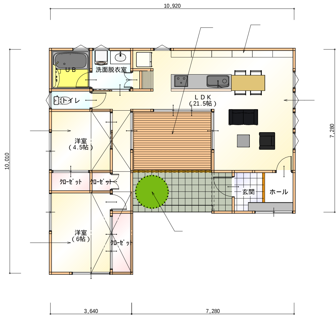
平面図
